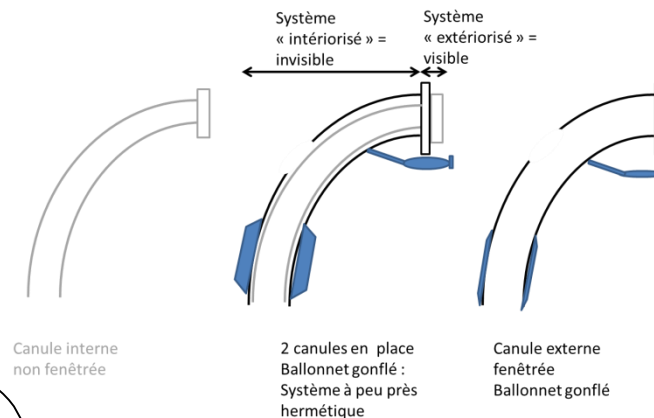
VUE DE PROFIL : CANULE INTERNE NON FENETREE
