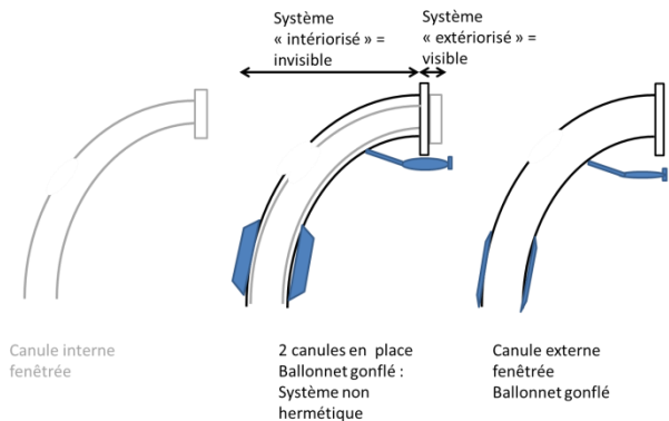
VUE DE PROFIL : CANULE INTERNE FENETREE
